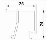
زهوار ۲ جداره ترمال
