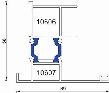
پروفیل واسط ۲ لنگه
