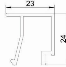
زهوار ۲ جداره ترمال
